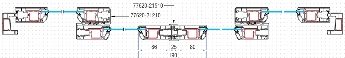
SEC A-A
