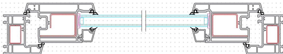
SEC A-A
