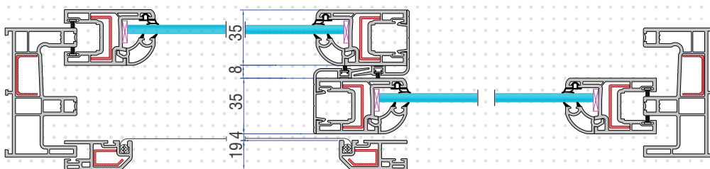
SEC A-A
