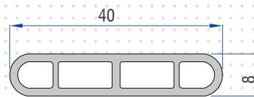
Louvre Blade 77390-20610
