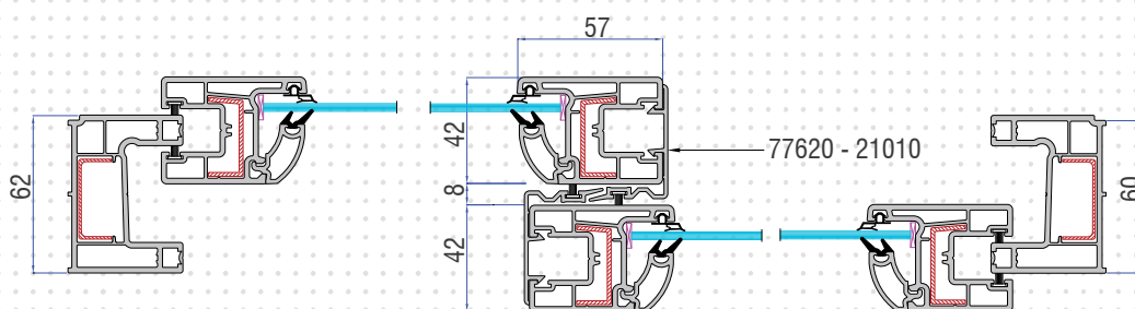
SEC A-A
