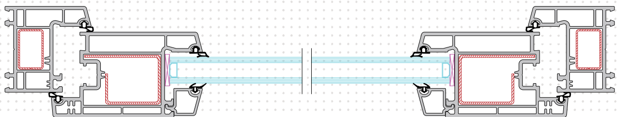
SEC A-A
