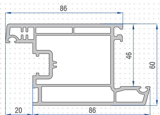
Inward Door Sash Profile 77601 - 12010
