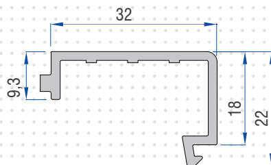
Louvre Clip 77390-20310
